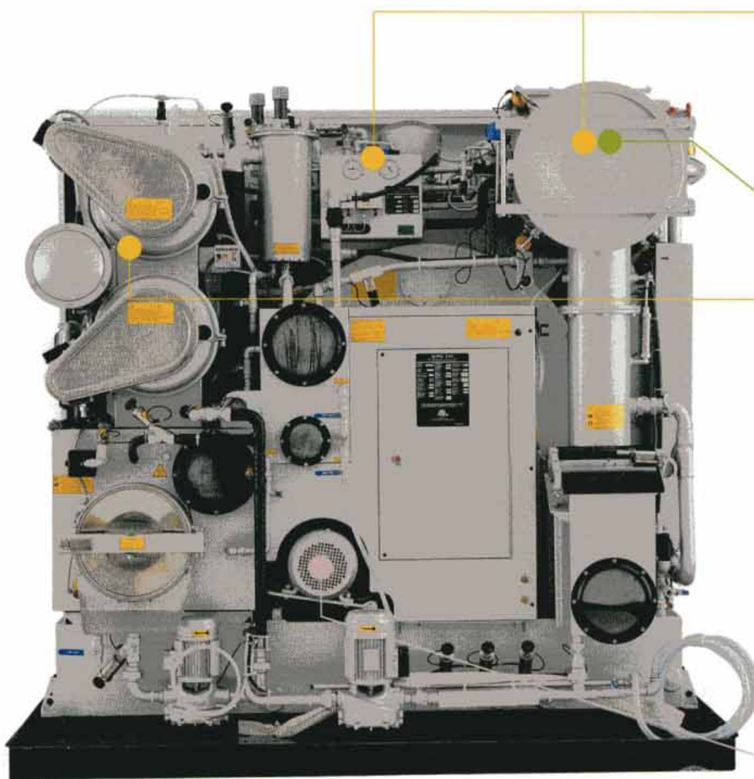
P440背面図
